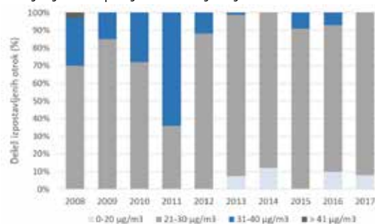
Slika 4: Izpostavljenost otrok (0-15 let) PM 10 v zunanjem zraku. Kazalniki okolja, ARSO.
